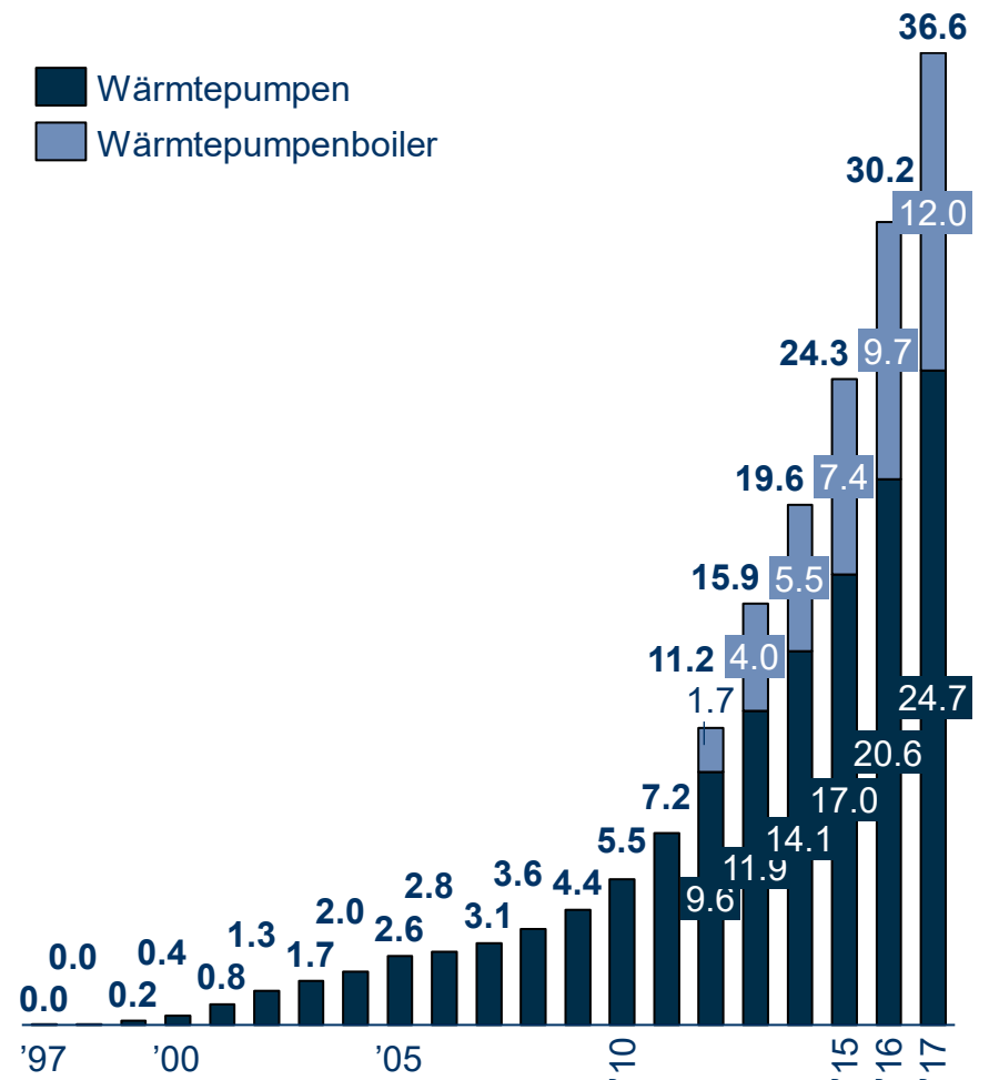
Anzahl der Wärmepumpen und Wärmepumpenboiler - Flandern, in Tsd. Einheiten, 1997–2017A -
